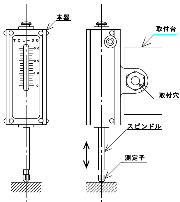
<図 2 > 取付図・各部名称
